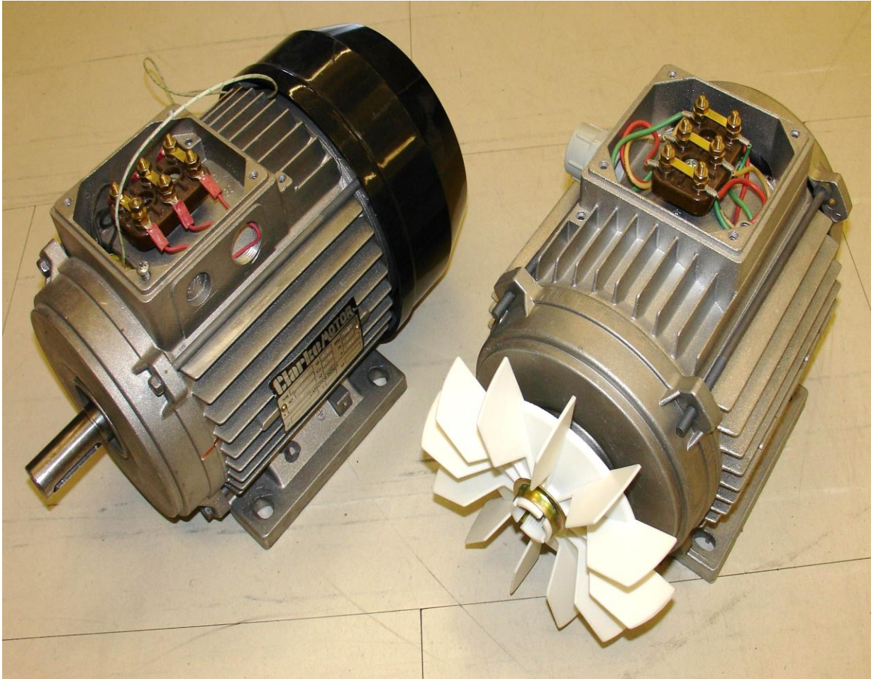
3- Phase SCIM
